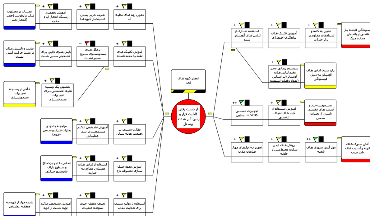
شکل ۵. تحلیل ریسک انفجار، کوره‌های ذوب
